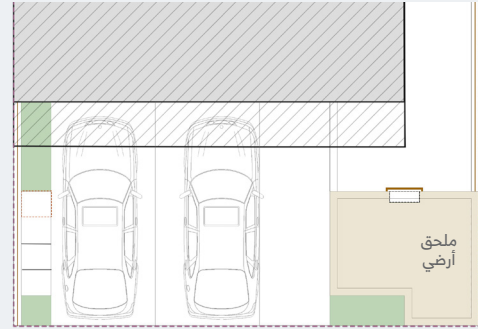
مسقط أفقي لموقع وحدة التكييف الخارجية
